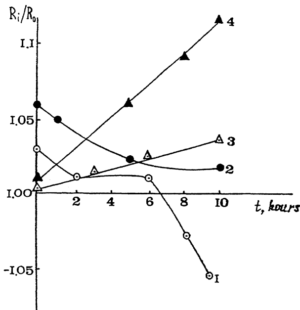
Рис. 1. Зависимость отношения ИОС R_i/R_0 от времени ИК облучения для образцов GaAs, легированных: 1, 2 — теллуром, 3, 4 — оловом. R_0 — значение ИОС для стехиометрического кристалла.
