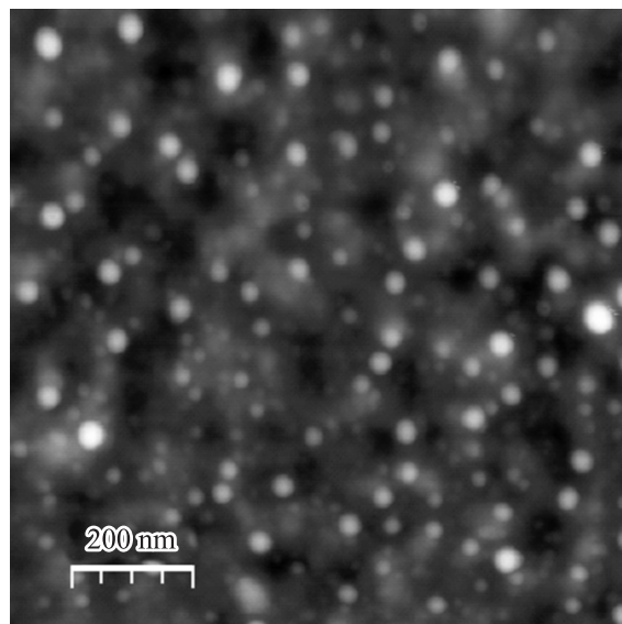
Рис. 1. AFM-изображение поверхности имплантированного ионами \text{Ag}^+ и отожженного образца \text{Cd}_x\text{Hg}_{1-x}\text{Te/CdZnTe} ( x \sim 0.223 ).
