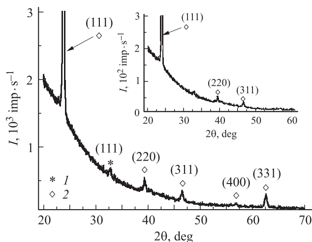
Рис. 2. GI XRD-спектр образца гетероструктуры \text{Cd}_x\text{Hg}_{1-x}\text{Te/CdZnTe} ( x \sim 0.223 ) после имплантации ионами \text{Ag}^+ . Глубина проникновения рентгеновского излучения < 200 \text{ nm} при \theta_{\text{inc}} = 1^\circ . 1 — \text{Cd}_{0.20}\text{Hg}_{0.80}\text{Te} , 2 — \text{Ag}_2\text{O} . На вставке — спектр рентгеновской дифракции образца в брэгговской конфигурации.
