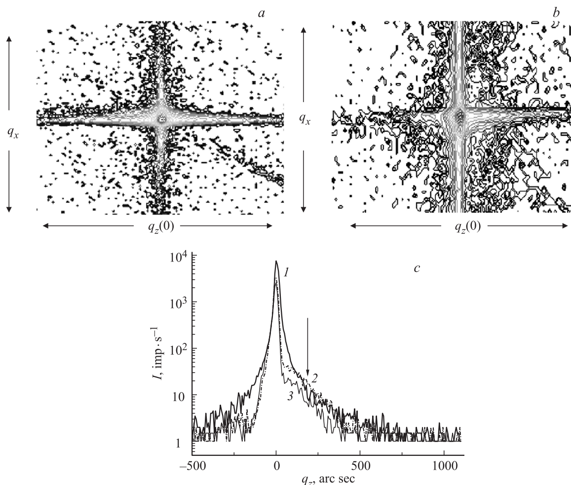
Рис. 3. Карты обратного пространства образца гетероструктуры \text{Cd}_x\text{Hg}_{1-x}\text{Te/CdZnTe} ( x \sim 0.223 ) до (a) и после (b) имплантации ионами \text{Ag}^+ , полученные из совместного \omega - и \omega-2\theta -сканирования с использованием высокоразрешающих модулей. c — распределение интенсивности диффузного рассеяния от образца вдоль вектора дифракции — направление q_z . 1 — исходное состояние образца, 2 — после имплантации \text{Ag}^+ , 3 — после отжига.
