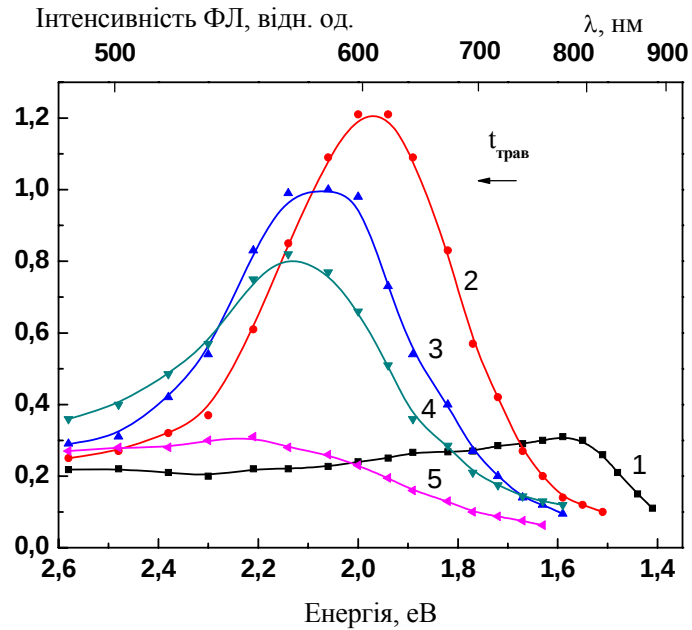
Рис. 1. Спектри фотолюмінесценції багатошарової структури (nc-Si-SiO_x-SiO_y)_n до (1) і після травлення у парі HF протягом 100 (2), 120 (3), 160 (4) та 200 (5) секунд. Товщини шарів SiO_x – по 3,5 нм, SiO_y – по 8,5 нм, n = 37 .
