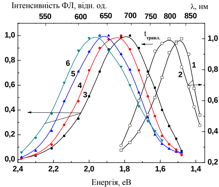
Рис. 2. Нормовані спектри фотолумінесценції багатошарової структури (nc-Si-SiO_x-SiO_y)_n до (1) і після травлення у парі HF протягом 25 (2), 110 (3), 140 (4), 190 (5) та 210 (6) секунд. Товщини шарів SiO_x – по 6 нм, SiO_y – по 13 нм, n = 31 .
