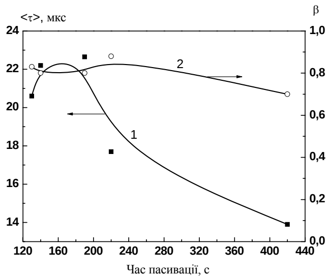
Рис. 7. Залежність середнього часу життя ФЛ (1) і параметра дисперсності β (2) від часу пасивації зразка серії 2.
