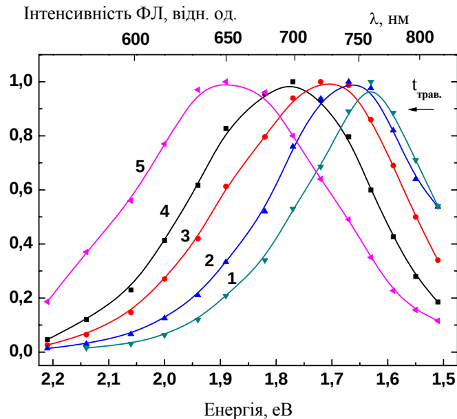
Рис. 3. Нормовані спектри фотолумінесценції багатошарової структури (nc-Si-SiO_x-SiO_y)_n після травлення у парі HF протягом 10 (1), 20 (2), 40 (3), 80 (4) та 120 (5) хвилин. Товщини шарів SiO_x – по 10 нм, SiO_y – по 25 нм, n = 37 .
